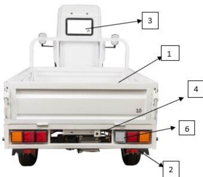
2 - THE OVERALL CAR – BACK – a jármű hátúlnézetből
